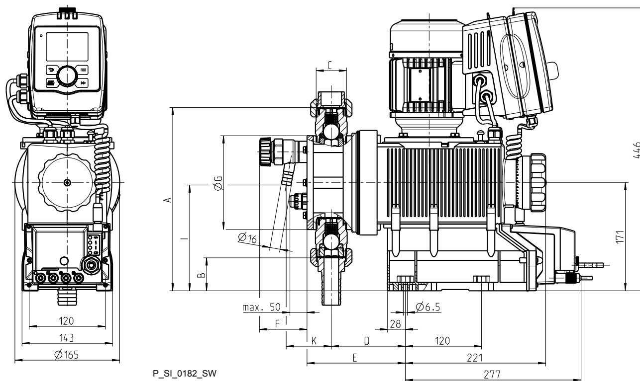
Fig. 2: Rappresentazione non strettamente vincolante - Misure in mm
