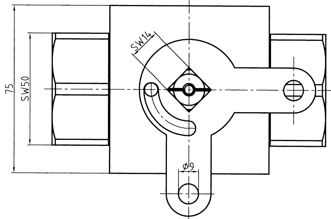
Ansicht ohne Handhebel
