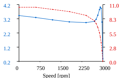
Torque [p.u.]
