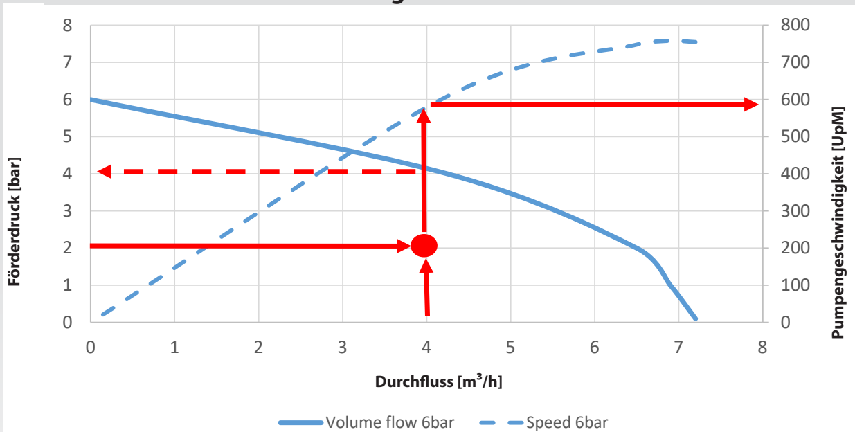
Leistungskurve EH25
