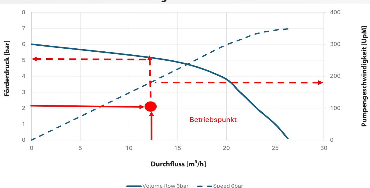
Leistungskurve EH50
