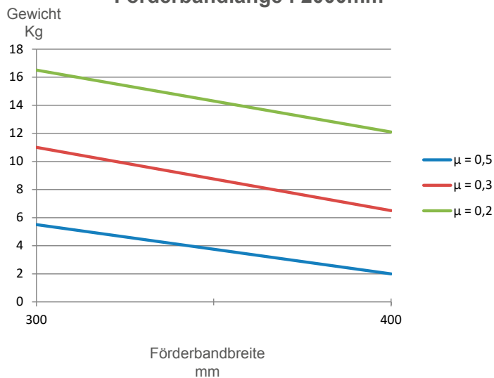
Förderbandlänge : 2000mm
