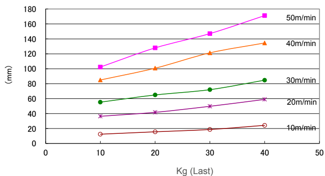
Bremsweg PM500FE 60m/min - Kartonage
