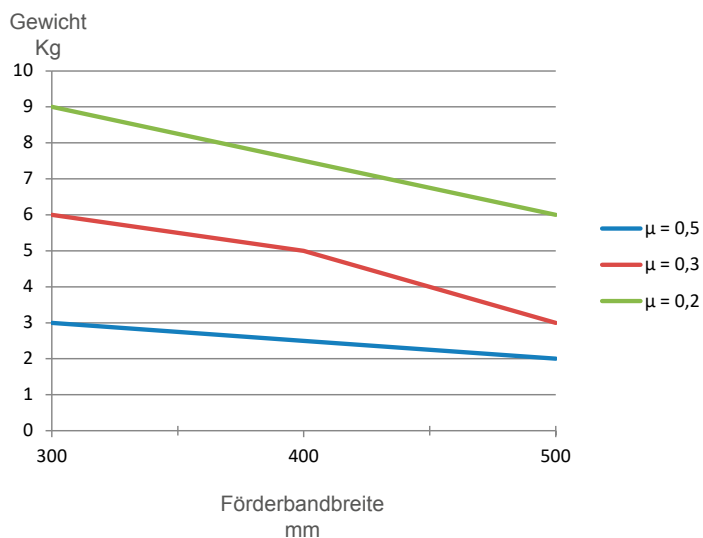
Förderbandlänge : 1500mm
