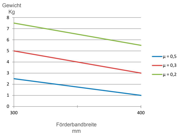
Förderbandlänge : 2000mm
