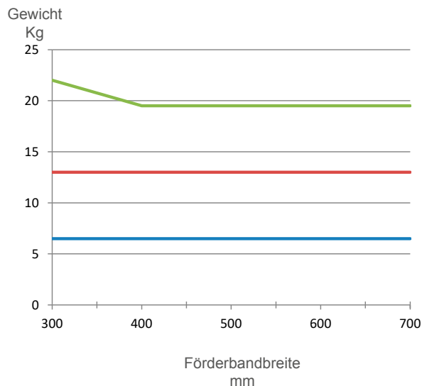
Förderbandlänge : 1500mm
