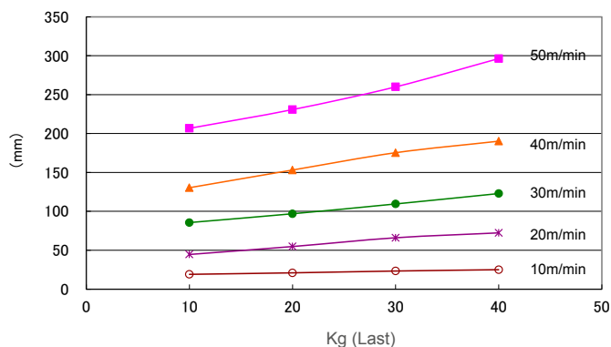
Bremsweg PM500FE 60m/min - Kunststoffkiste
