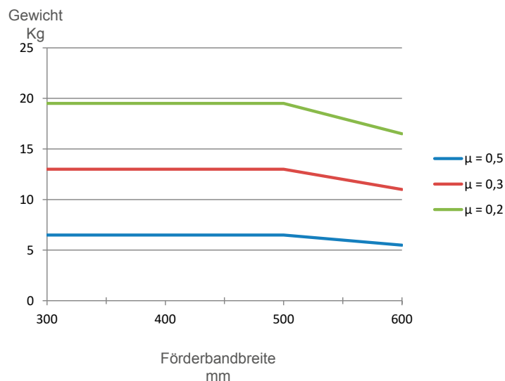
Förderbandlänge : 2000mm
