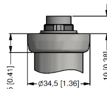
Binder Serie 723, 5-pin (IP 67)
