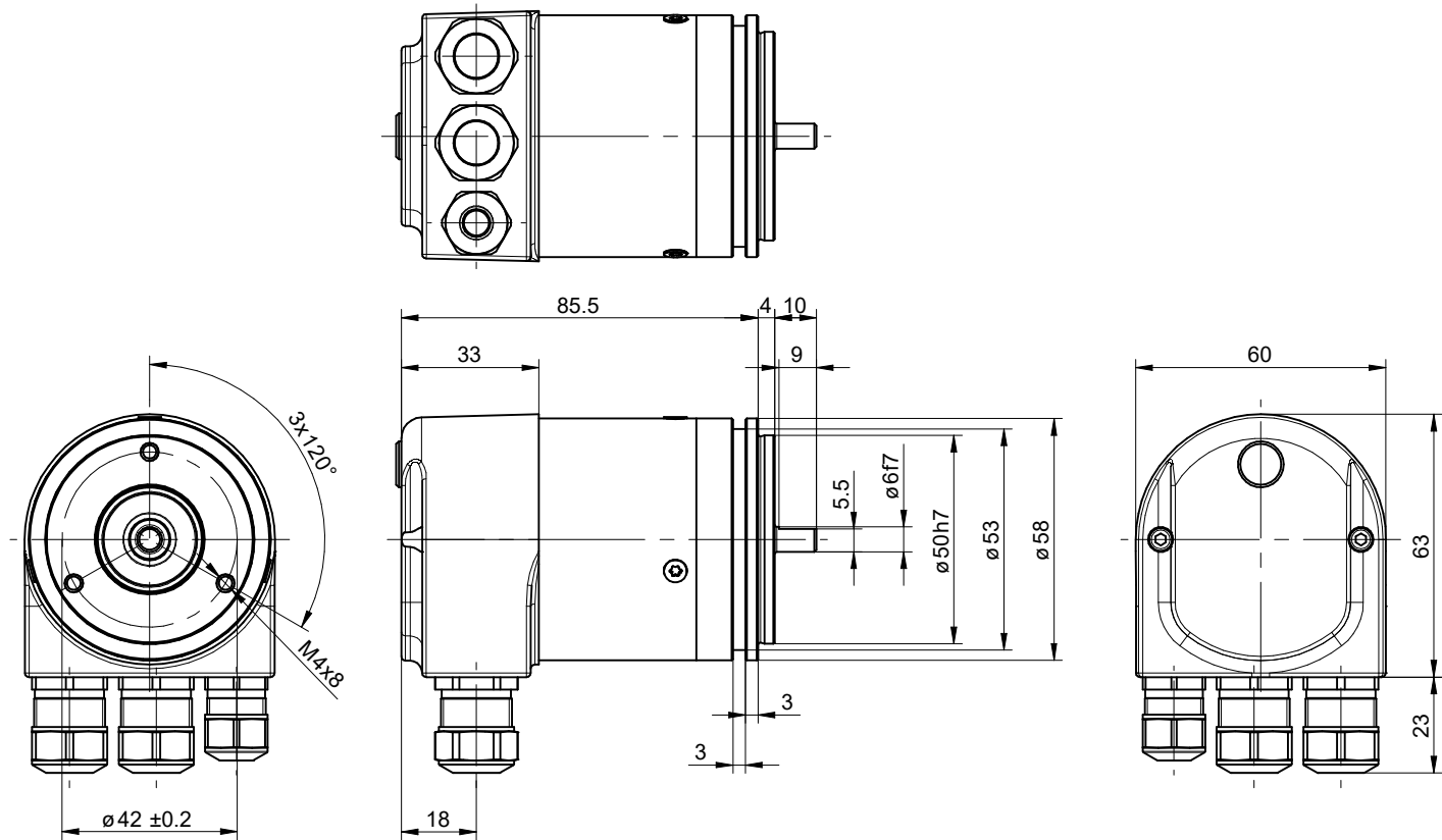
EN580C.ML-SU - Kabelverschraubung
