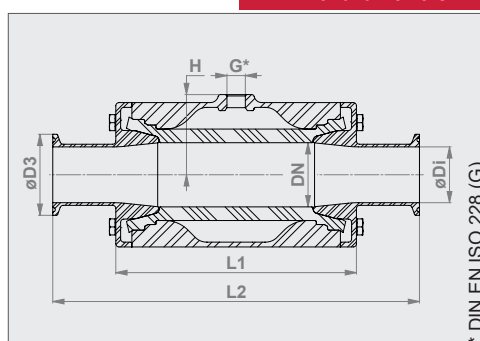
Exempl. Ansicht / Exempl. view (DN 65 – DN 100)
