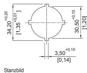
Stanzbild
