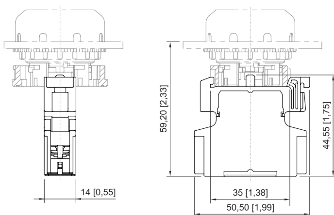
Kontaktelement für Fronteinbau
