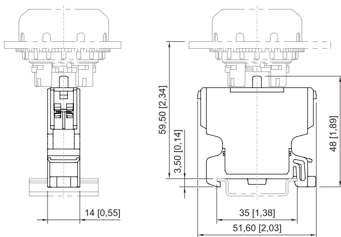
Kontaktelement für Tragschienenmontage
