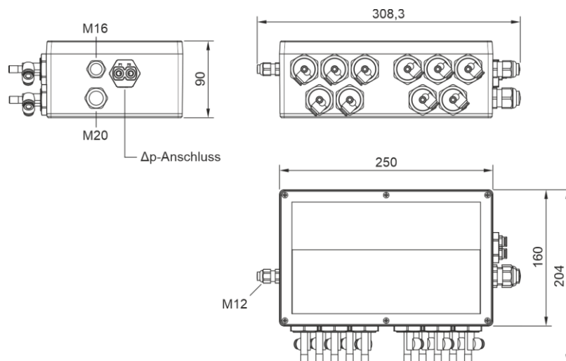
Bild 9: Maße ESM-12 DP 10V IECEx
