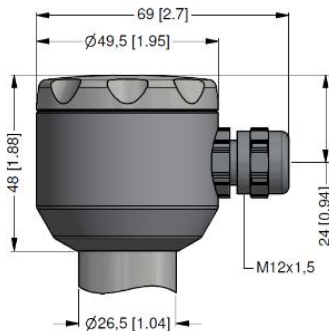
Kompakt-Feldgehäuse (IP 67)
