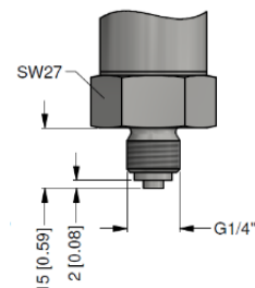
G1/4" EN 837
