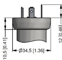
ISO 4400 (IP 65)
