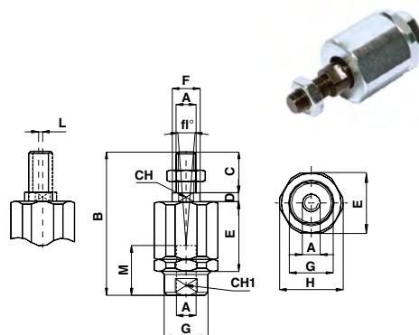
KF-22 EMBOUT ROTULÉ OSCILLANT D'ÉQUERRE
