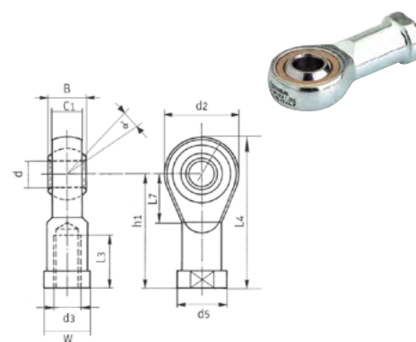
NW COMPENSATEUR D'ALIGNEMENT
