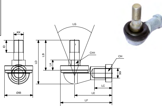
KF-22 EMBOUT ROTULÉ OSCILLANT D'ÉQUERRE
