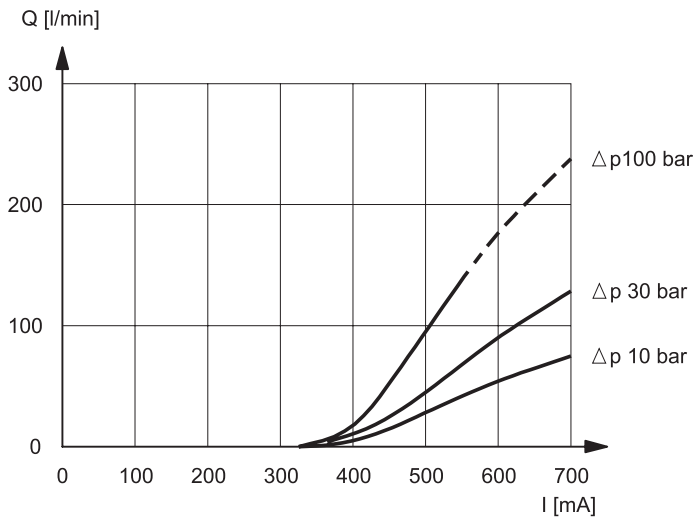
SPOOL TYPE 91
