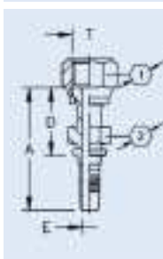
Skive Nipple
