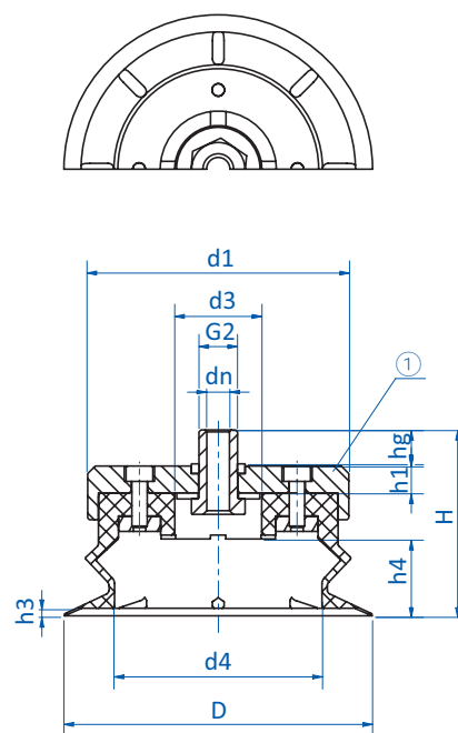
Zeichnung D
