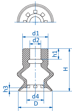
Zeichnung A
