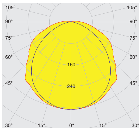
cd/klm 100% — C0 - C180 — C90 - C270 typisch mit Diffusor, klare Leuchtenwanne
