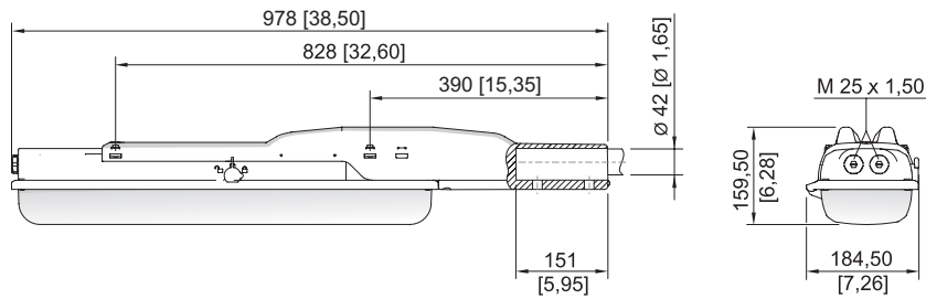
Baugröße 2
