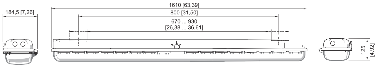
Baugröße 6
