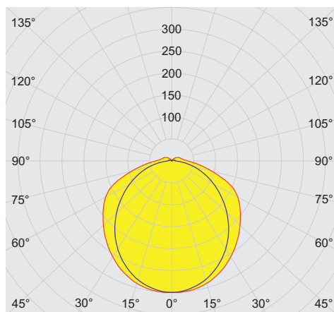
cd/klm 100% — C0 - C180 — C90 - C270 typisch ohne Diffusor, diffuse Leuchtenwanne
