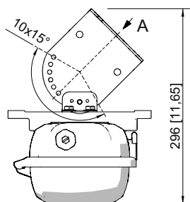
Montageschiene
