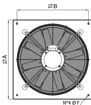
QCM-ATEX 630-710
