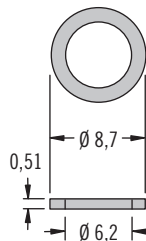
Arruela lisa
