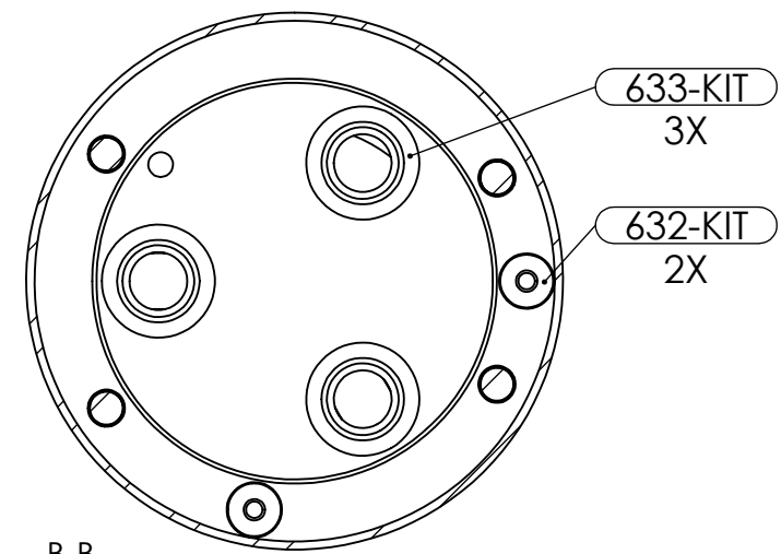
B-B
