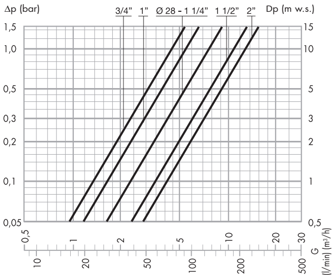
Empfohlene DURCHFLUSSMENGEN für einen stabilen Betrieb und eine Präzision von ±2°C (abgeglichene Drücke Warm/Kalt)
