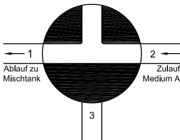
3-Wege-Kugelhahn mit T-Bohrung
