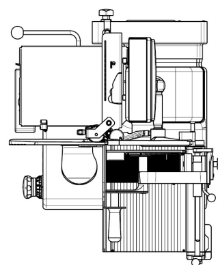
VSP F 10" Display Draufsicht
