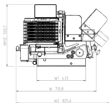
VSP F 7" Display Frontansicht
