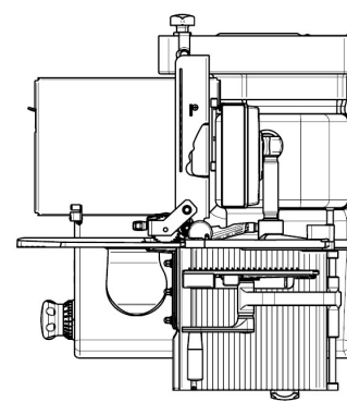
VSP F 7" Display Draufsicht
