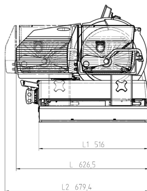
VSP F 7" Display Seitenansicht
