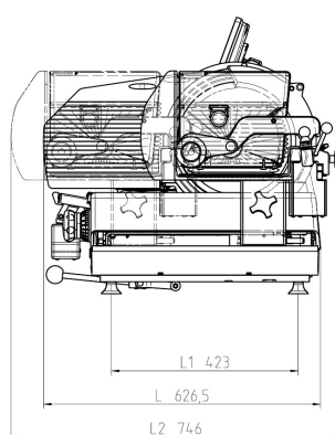
VSP F 10" Display Seitenansicht
