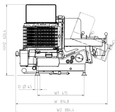
VSP F 10" Display Frontansicht
