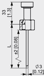
M01 | FLEXadapt ESF G3/8" Überwurfmutter, \varnothing 3 mm, gefedert
