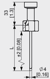
M04 | Sensor G3/8" Überwurfmutter, \varnothing 4 mm, gefedert
