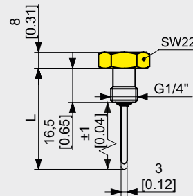
G03 | Gewinde G1/4" \varnothing 3 mm, gefedert
