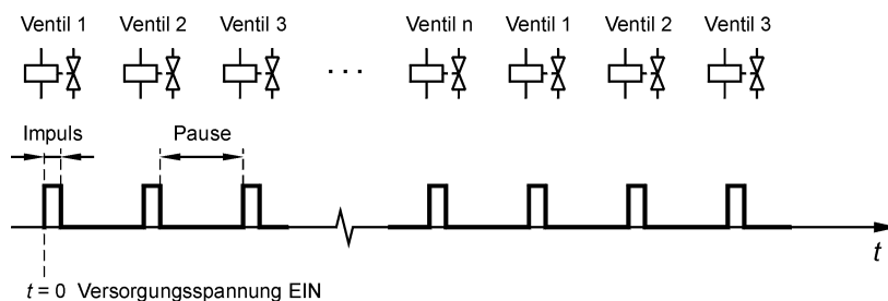
Bild 10: Fortwährende Abreinigung bei Einstellung des Parameters 05 auf den Wert 0
