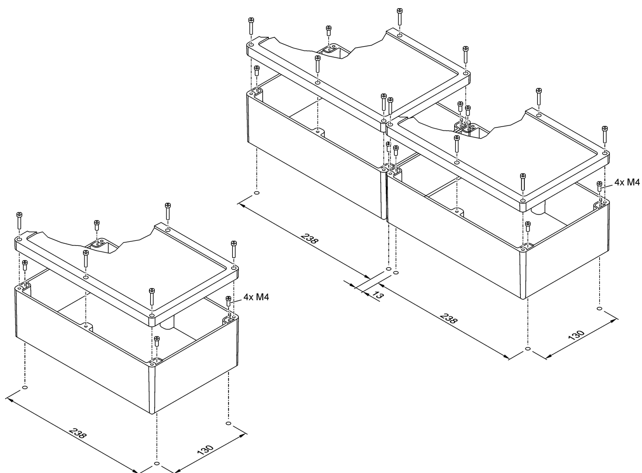
Bild 4: Gehäuse-Montage
