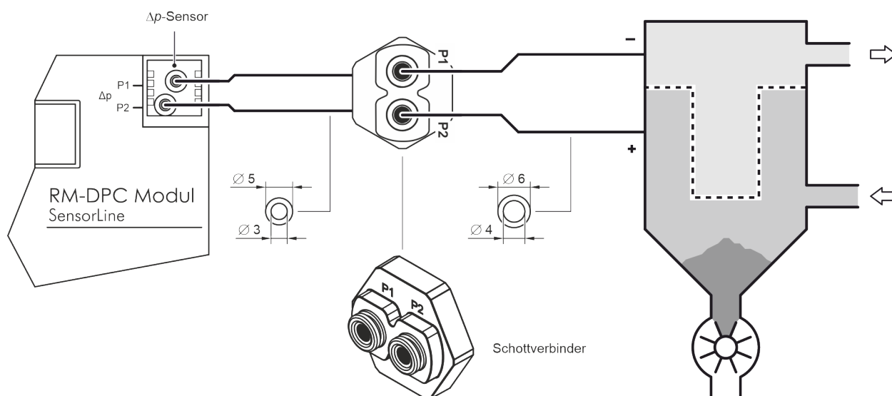
Bild 7: Anschluss der Differenzdruck-Messleitungen
