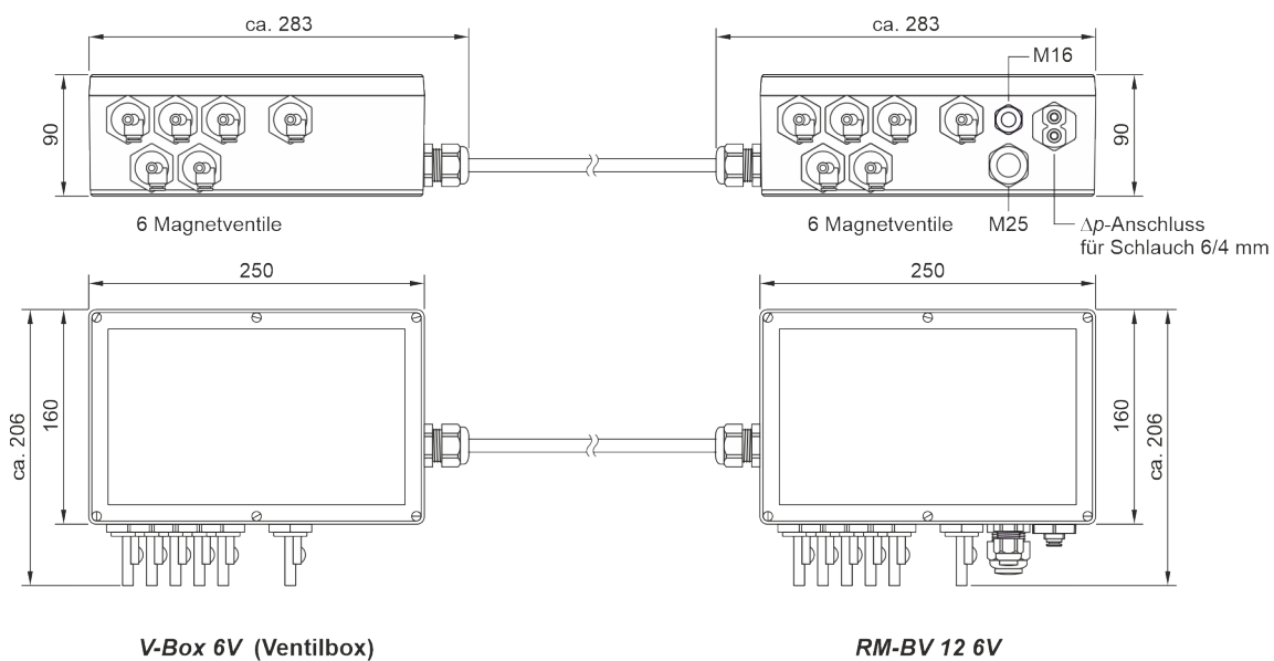
Bild 3: RM-BV 12 6V mit separater Ventilbox V-Box 6V
