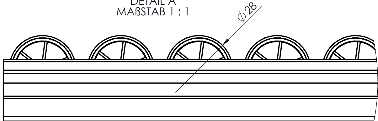
DETAIL B MAßSTAB 1 : 1
