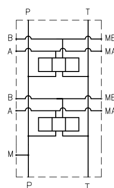
Schema idraulico in parallelo
