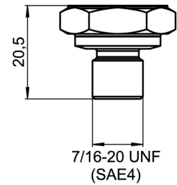
7/16-20 UNF mit O-Ring (SAE 4) (BCID: U02)
