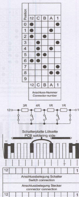
Code 731 BCD positiv + Komplement - kurzschliessend
