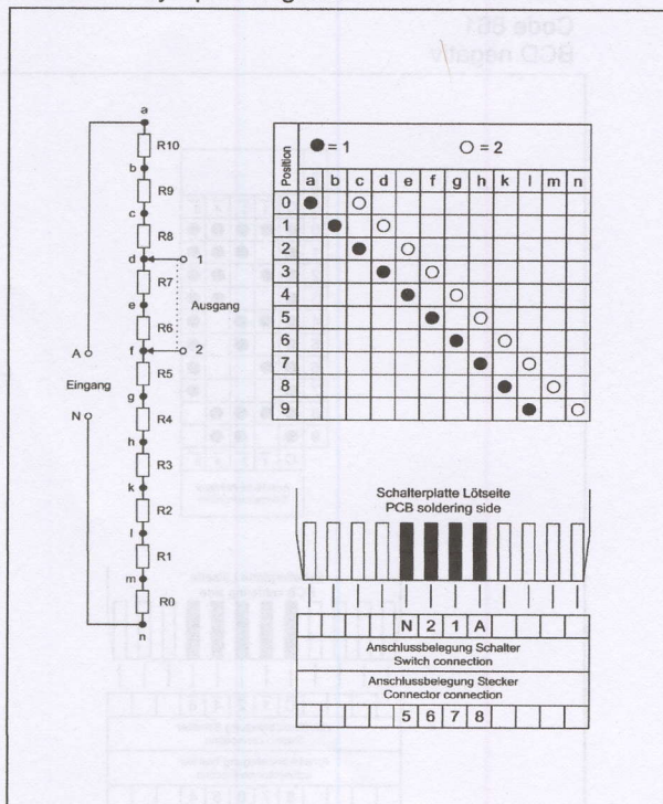
Code 618 Kelvin Varley Spannungsteiler
