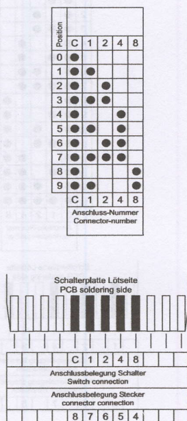
Code 731 BCD positiv + Komplement - kurzschliessend
