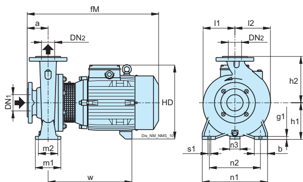
Flanges EN 1092-2
