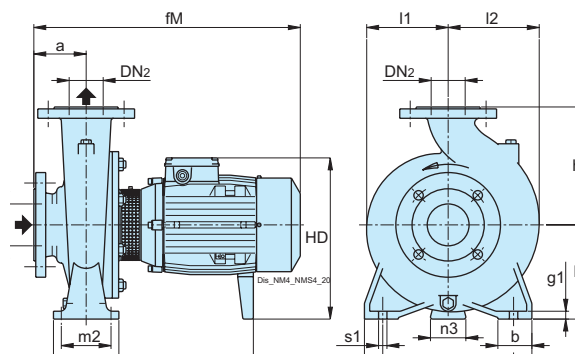
Flanges EN 1092-2
