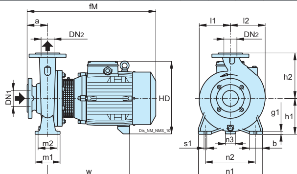
Flanges EN 1092-2
