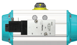
Elettrovalvola
