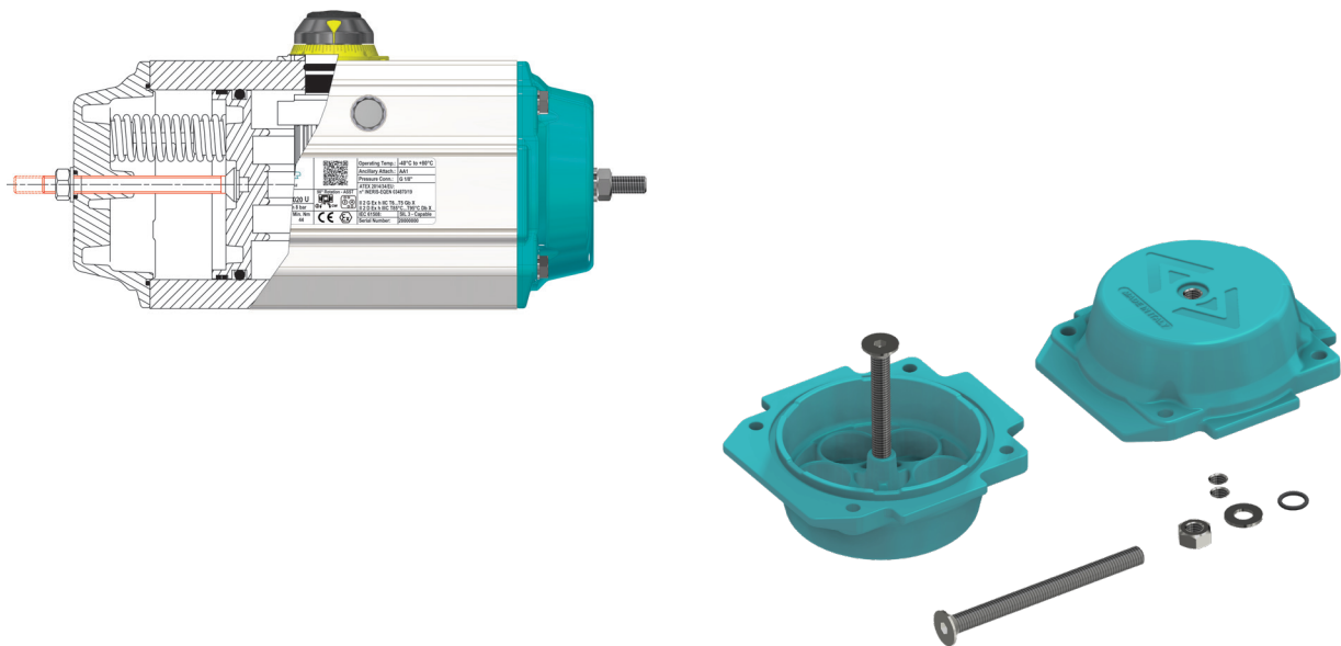
Viti lunghe per regolazione corsa a 0 \div 90^\circ
