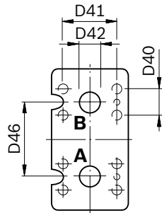
Teilansicht Y
