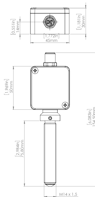
Einschraubvariante M14x1,5 lang (1-Kanal) -40 °C ... +150 °C [-40 °F ... +302 °F]
