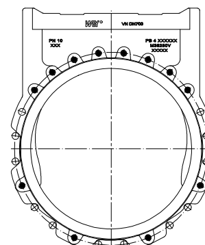
DN 700+800
