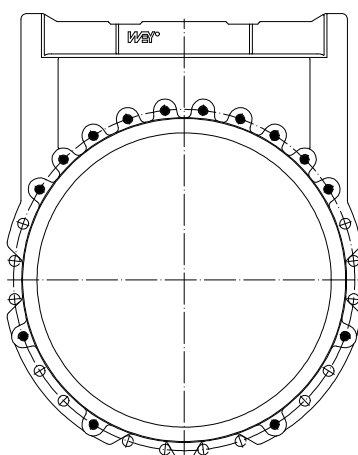
DN 900-1000
