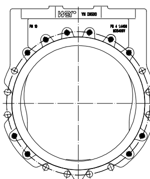
DN 450-600
