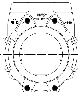
DN 65-200
