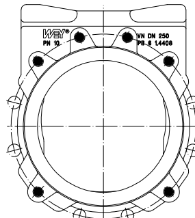
DN 250+300
