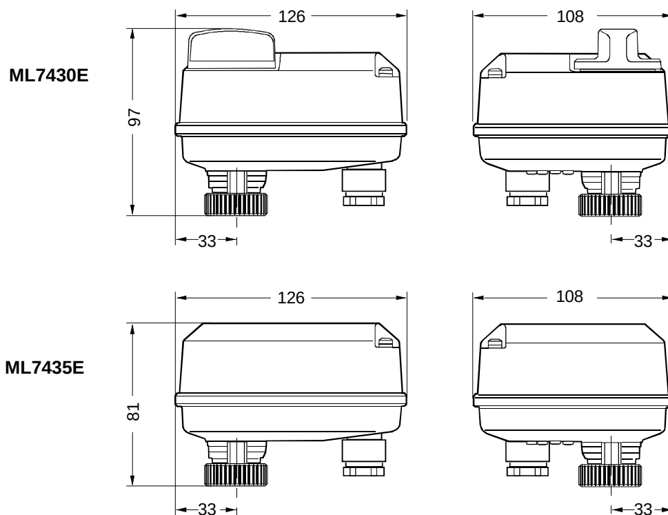
Fig. 2 Dimensioni in mm
