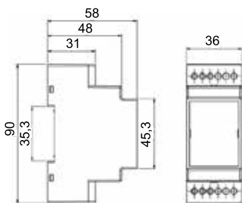
Dimensions(mm)Type PK 25)
