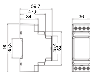
Dimensions(mm)Type PK 28)
