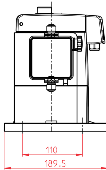
EcoPro Seitenansicht
