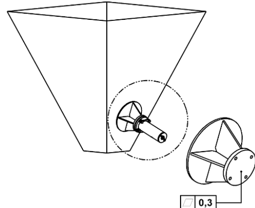
Anschweißbock, rund
