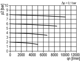
Durchflussdiagramm
