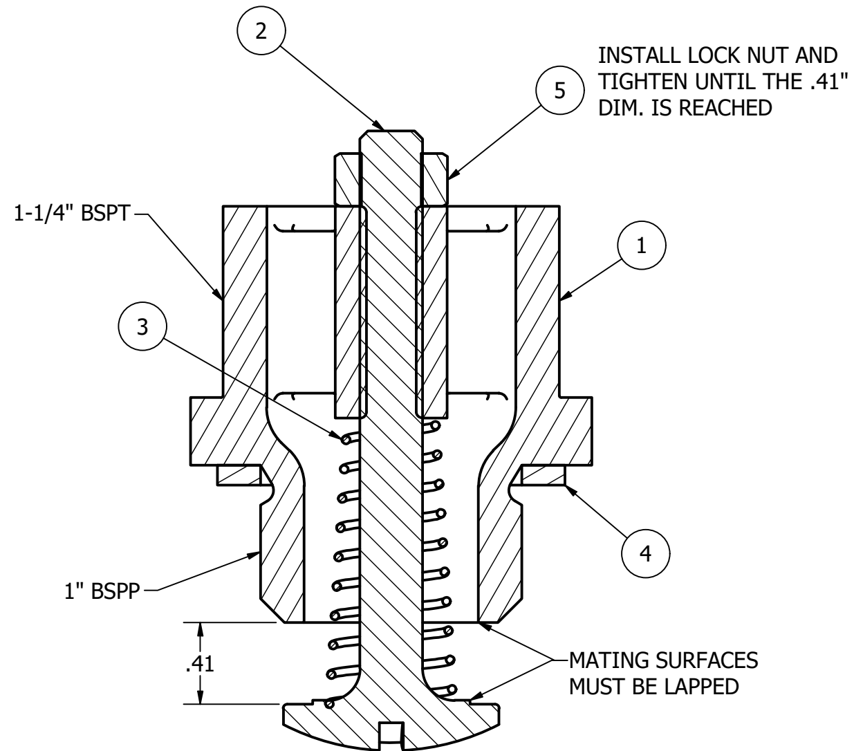
SECTION A-A
