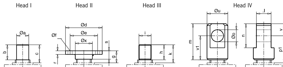
Design „A“
