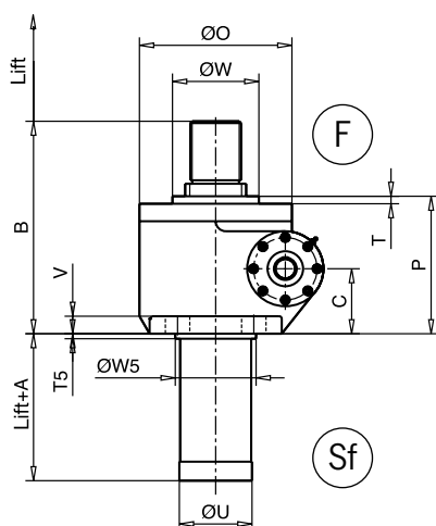
Design „A“
