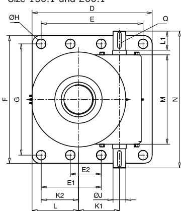
Size 150.1 und 200.1
