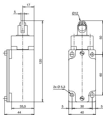
XCK-J 567 H29
