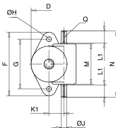
Size 0,5
