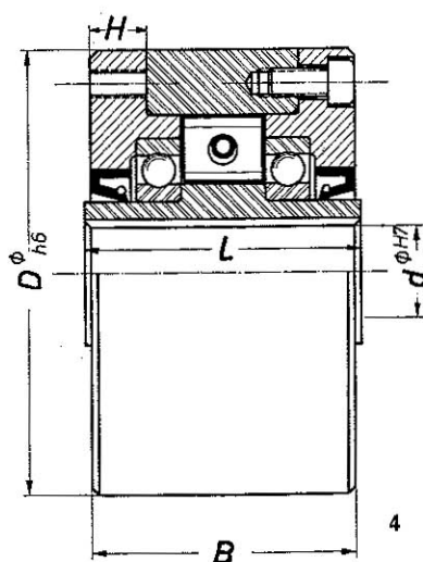
Séries FK, Dimensions 12-24
