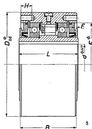
Séries FK, Dimensions 27-62
