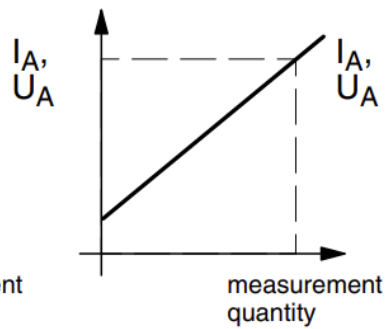
"live zero"
