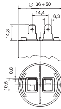
Fig. 1 Doppio Faston 6,35 x 0,8 mm
