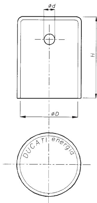
Fig. 9 Cappellotto. Fig. 9 Protective cap.
