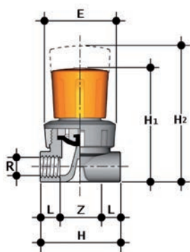
VMFV Minivalvola a membrana con attacchi femmina, filettatura cilindrica gas
