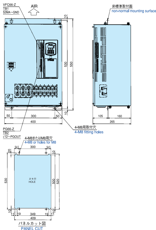
非標準タイプ (発熱部の外部分離型)
