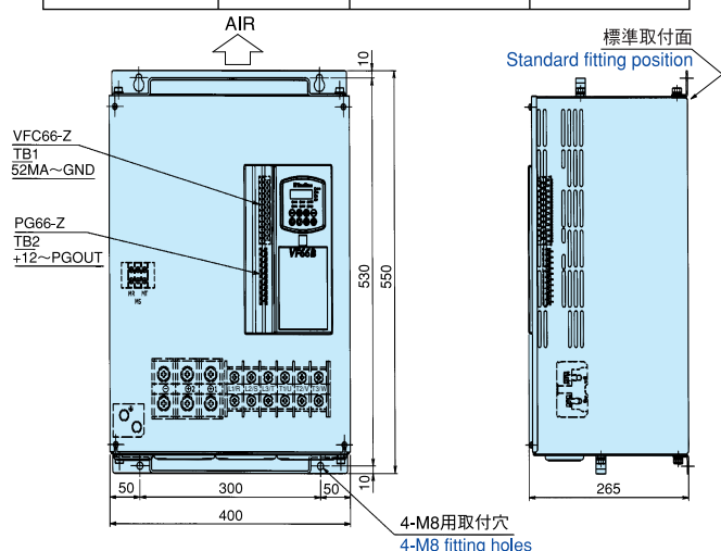
非標準タイプ (発熱部の外部分離型)
