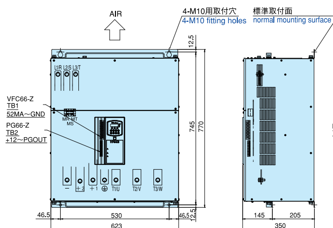
非標準タイプ（発熱部の外部分離型）
