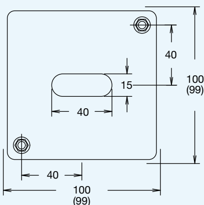
Bild 2: Einbaumaße und Strahlerabmessungen ( ) in mm
