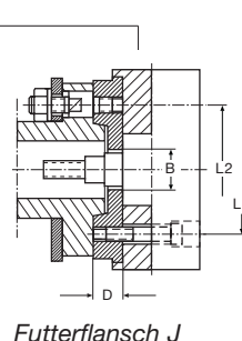
Futterflansch J
