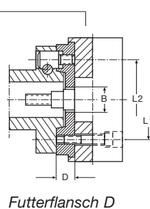
Futterflansch D
