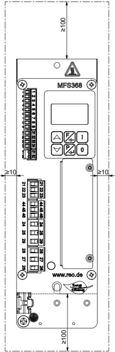
Einbauabstände
