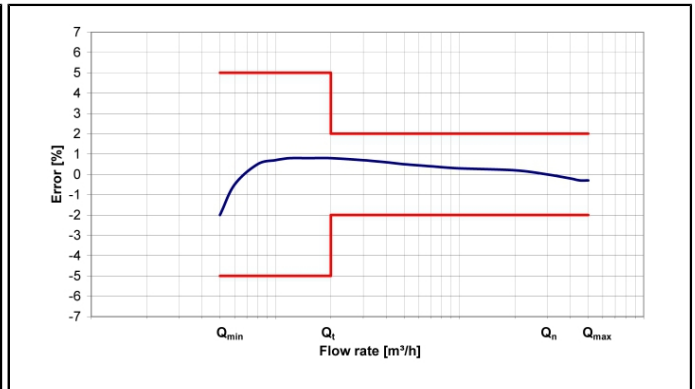
Typische Fehlerkurve
