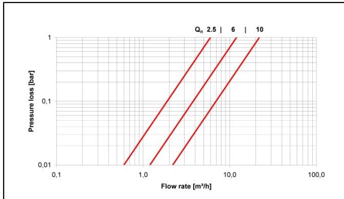
Druckverlust
