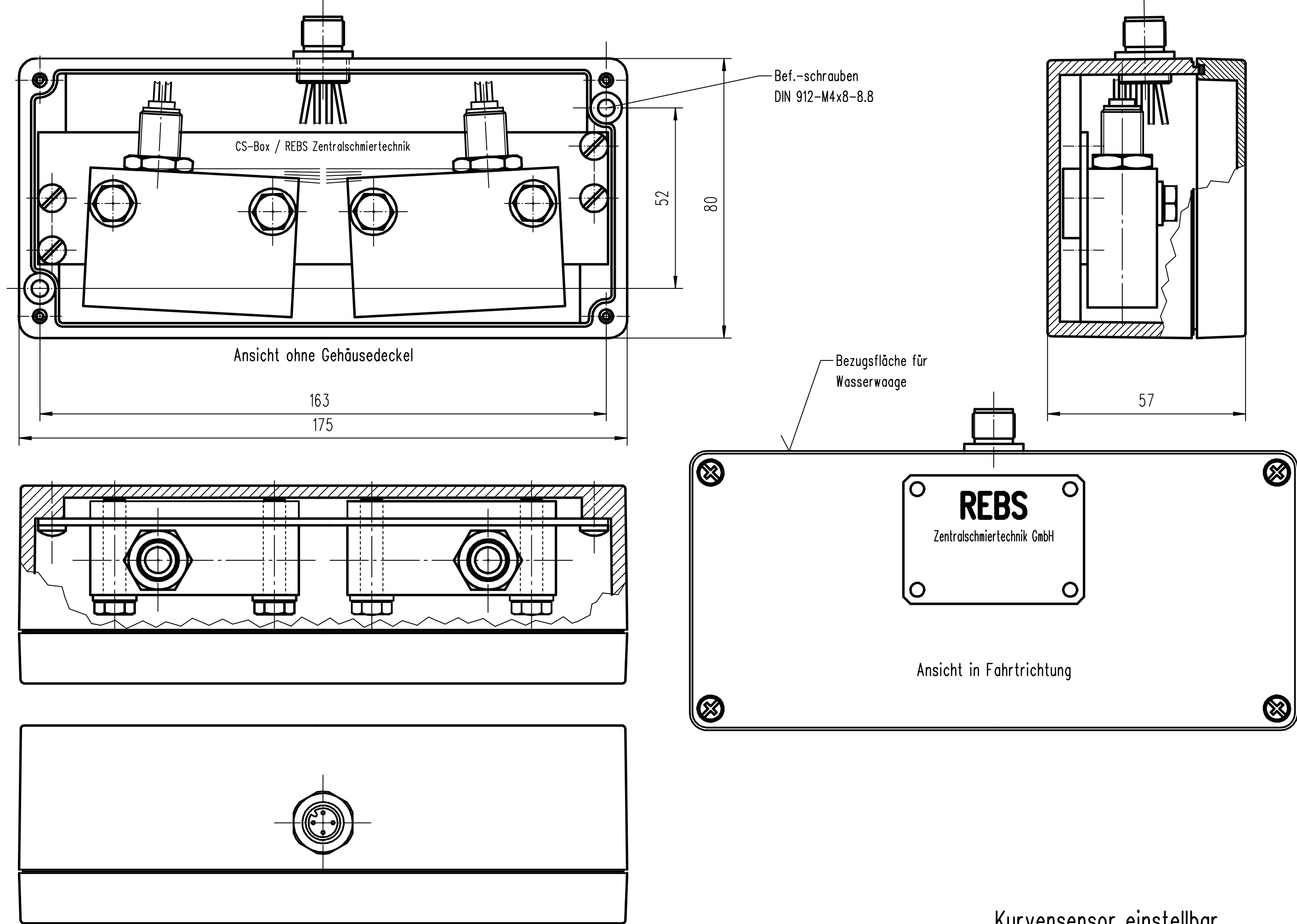
Kurvensor einstellbar CS-Box
